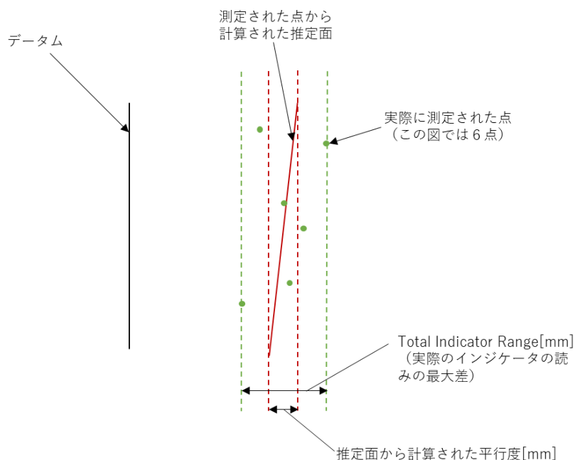
図4. 座標測定機により出力される平行度の考え方
